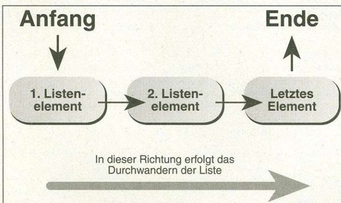
Einfach verkettete Liste: So sieht in der Regel intern der Aufbau oft benötigter dynamischer Datenstrukturen aus
